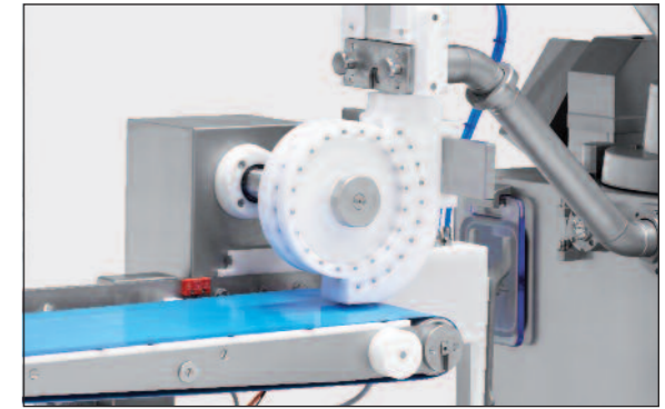
Formage de steaks hachés à l'aide de la guillotine et de la bande de formage
